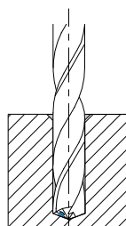
FASE 3 Foratura profonda senza passaggio misurabile rispetto al foro pilota
