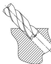
Fase 2: foratura profonda inclinata Utensile: punta elicoidale
