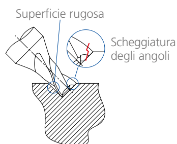
Fase 1: lamatura con fresa frontale lunga Utensile: fresa
