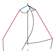
■ Smusso 60° ■ Angolo di punta 130°
