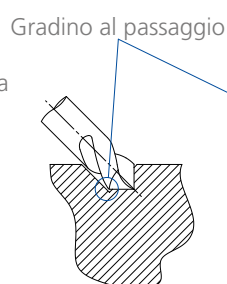
Fase 2: centratura Utensile: centrino NC
