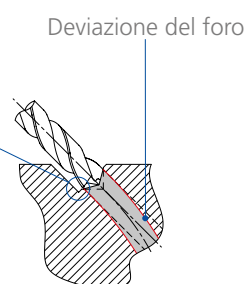
Fase 3: foratura inclinata Utensile: punta elicoidale
