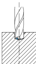
FASE 2 Punta guidata nel foro pilota
